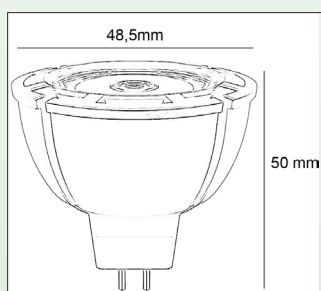
Lampans mått
